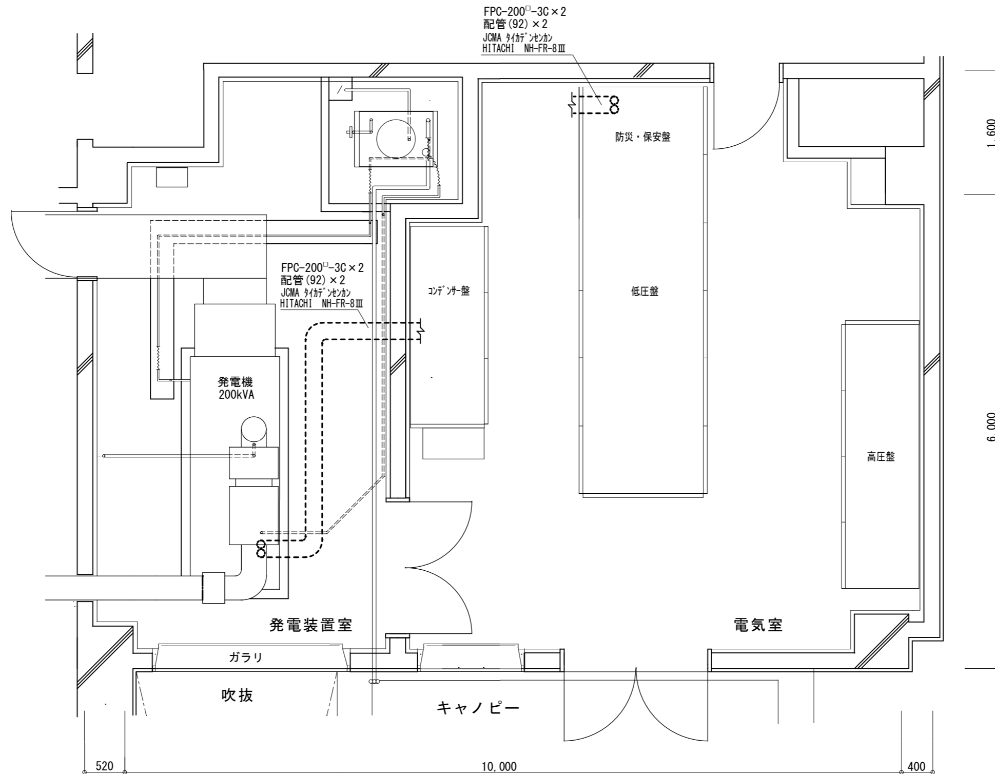
平面図（発電装置室・電気室）
