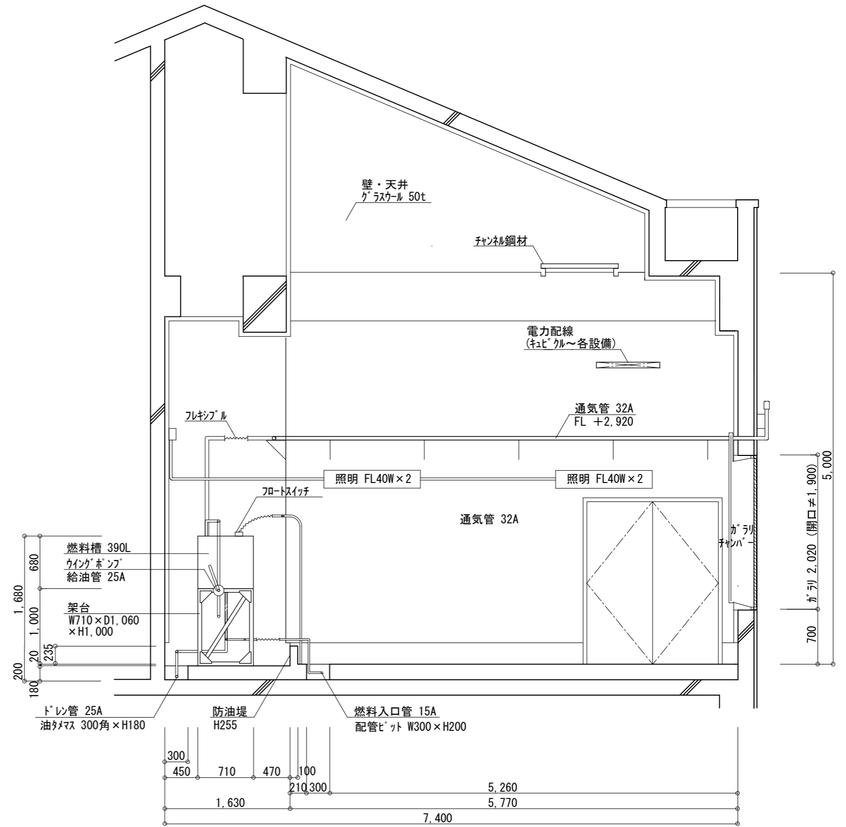
C展開図
