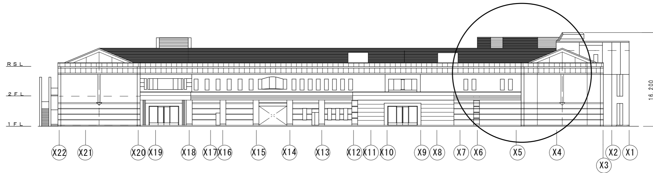
A 立面図
