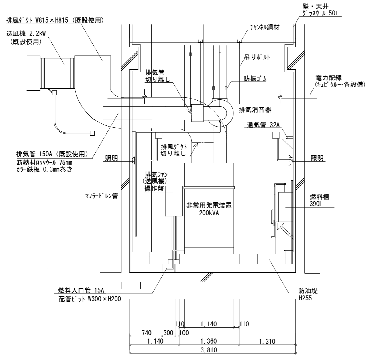
B展開図
